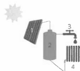
1. Zonnecollector | 2. Opslagvat zon-afw-er | 3. Sanitair warm water | 4. Afgifteenent voor ruimteverwarming (radiator)
